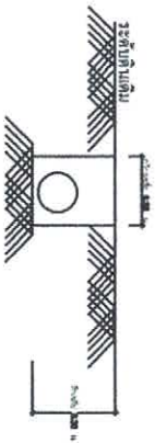
DETAIL งานชุดฝังท่อประปา PVC
